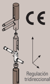
Detalle Bisagra
