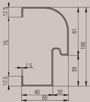
Modelo CR8
