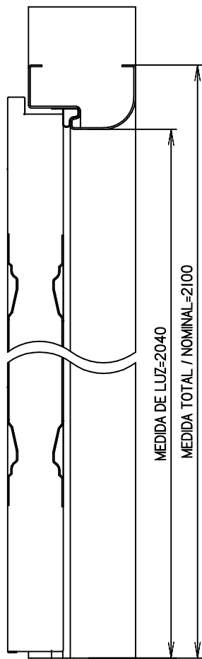
CORTE D-D 1:5
